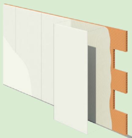
Tabiquería de ladrillo hueco gran formato con revestimiento de placa de yeso laminado (Muralit)
